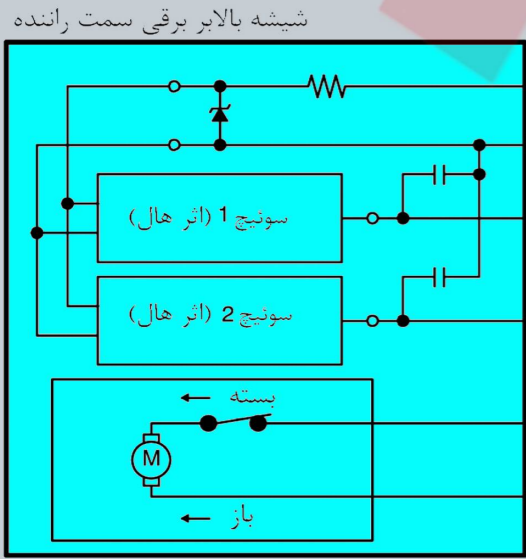
0912-201 سوییچ اصلی شیشه بالابر برقی
