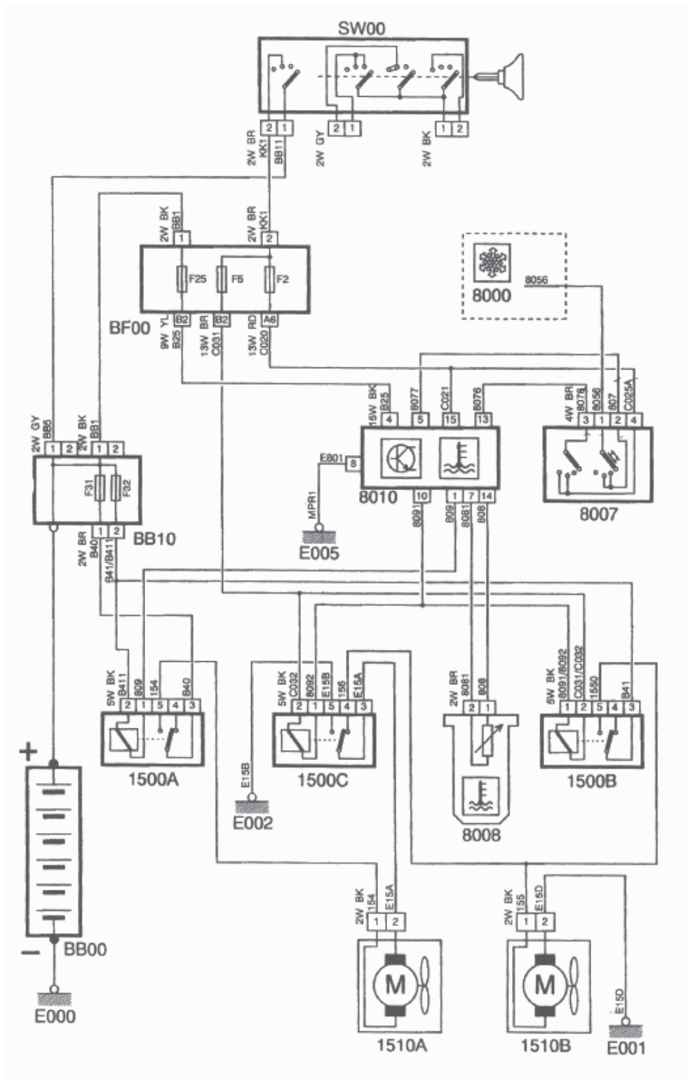
نقشه شماتیک مدار سیستم خنک کننده با کنترل یونیت فن
