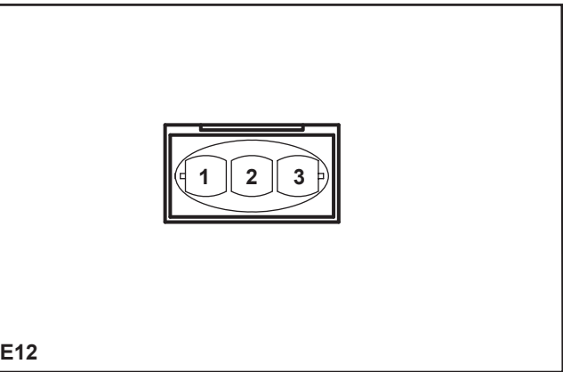
E12 Pin Definition
